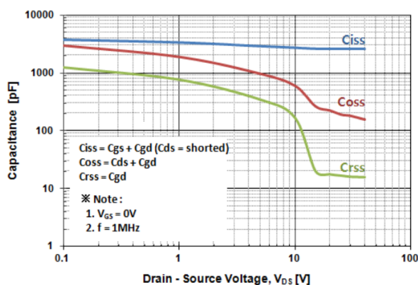
Fig. 5 Capacitance - V_{DS}
